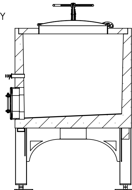
SECTION A-A SCALE 1 : 32
